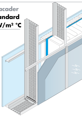
Bærende facader U-værdier, standard ned til 0,13 W/m 2 °C eller bedre
