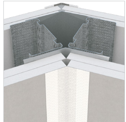
Variabel innerhörn
