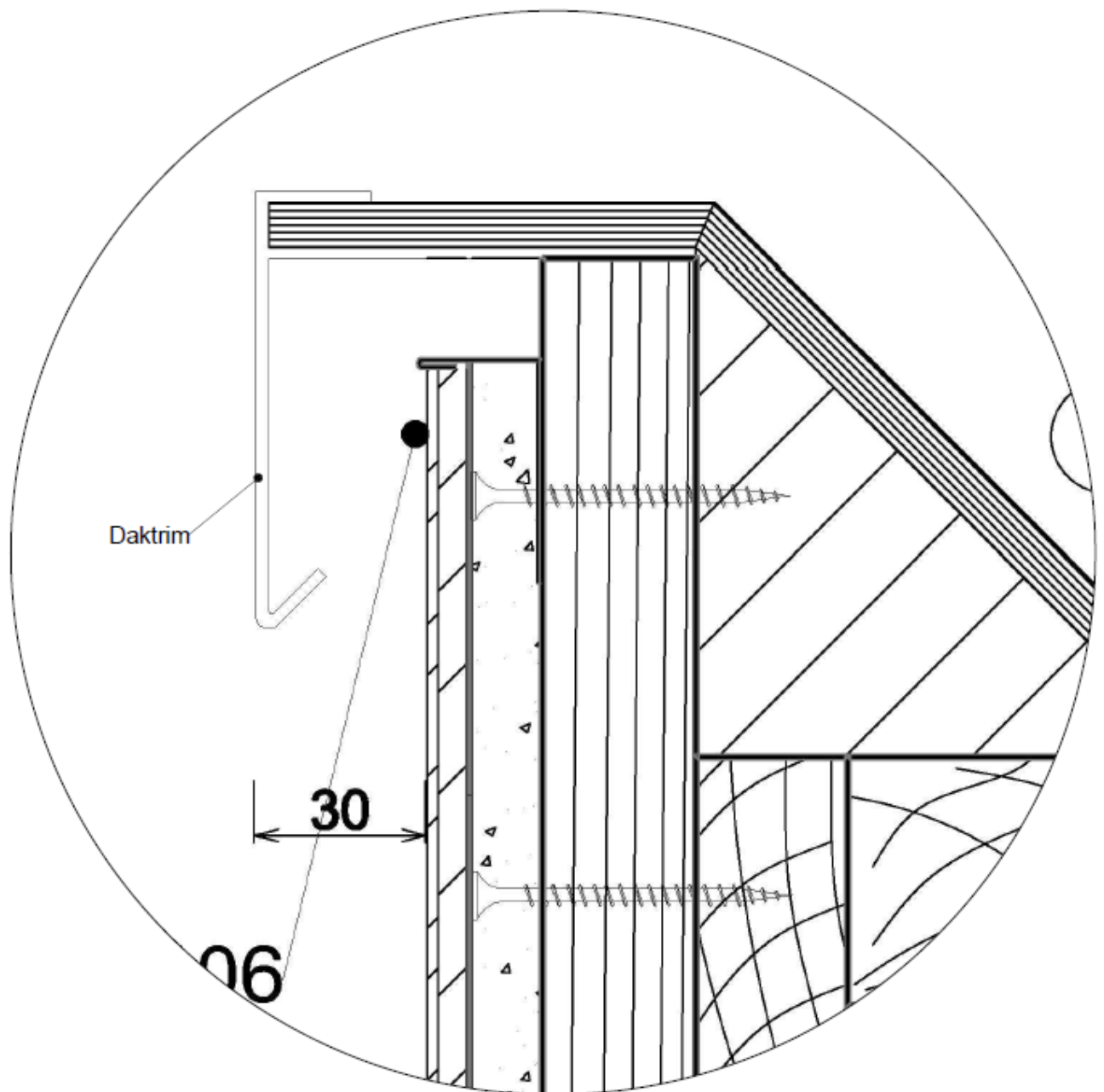
Geventileerd systeem - Bovenaansluiting / platdak beëindiging
