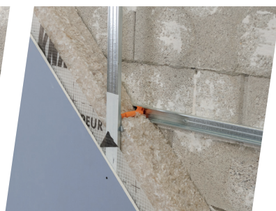
Le pose du pare-vapeur est obligatoire. Sa valeur Sd doit être >18 m en climat de plaine et > 57 m en climat de montagne.
