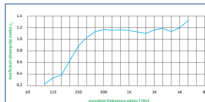
Graf prikazuje odvisnosti merjenega koeficienta absorpcije \alpha_s v odvisnosti od frekvenčnega spektra za mineralno volno z upornostjo zračnemu toku 5 kPa·s/m² pri debelini 75 mm.
