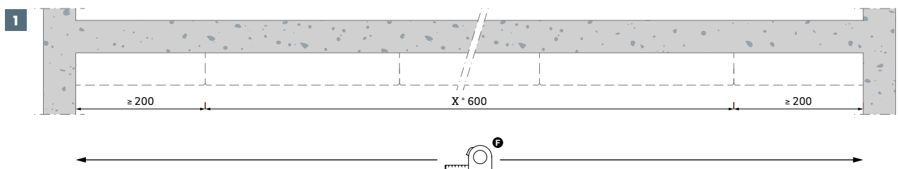
Onderaanzicht plafond
