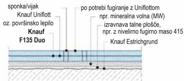
F135-V2 Stik plošč
