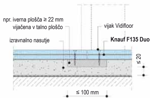
F135-V6 Stik elementov pri vratih
