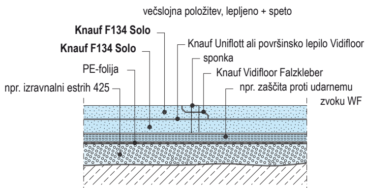
F134-V6 Stik elementov 2-slojno položen F 134
