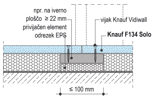
F134-V3 Elementi v območju vrat z EPS
