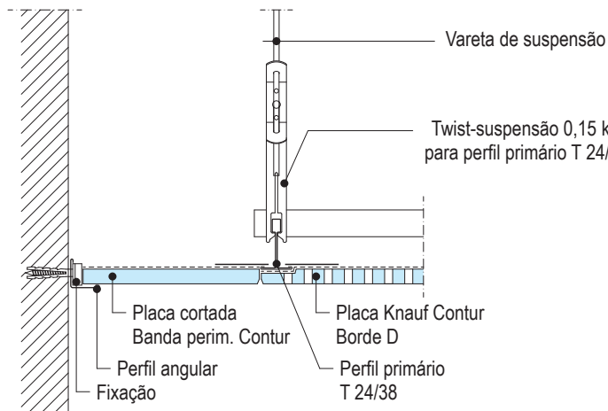
D147.pt-A1 Banda perimetral com angular paralelo ao perfil
