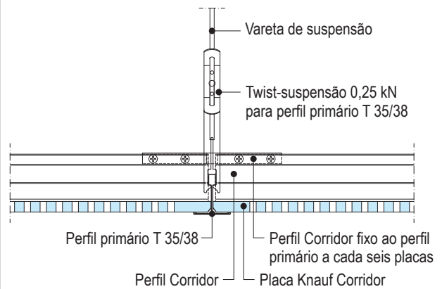
D148.pt-A6 Emenda do teto para comprimentos ≥ 2400 mm
