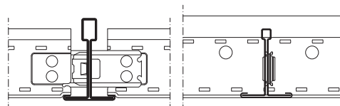
Perfil secundário T 24/32 (15/34) comprimento 1200 mm
