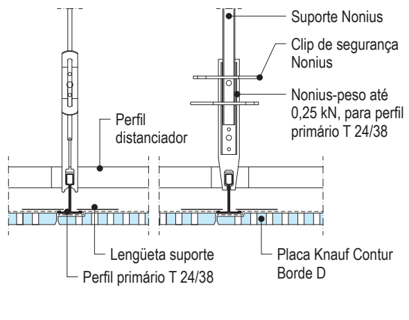
D147.pt-B1 Encontro entre as placas e o perfil de suporte
