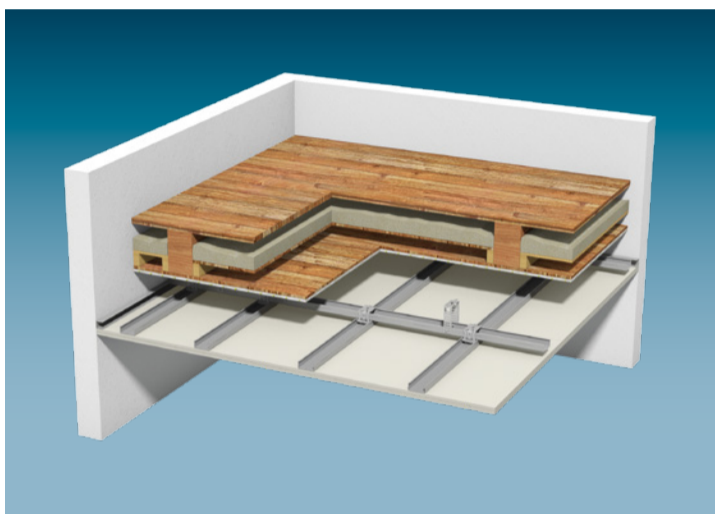
Eine der 14 verschiedenen Holzdeckenarten, die entscheidend für die Konstruktion sind.
