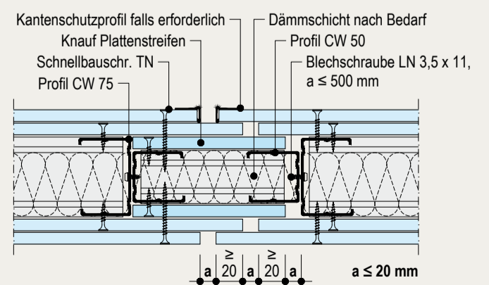
Bewegungsfuge mit Brandschutz
