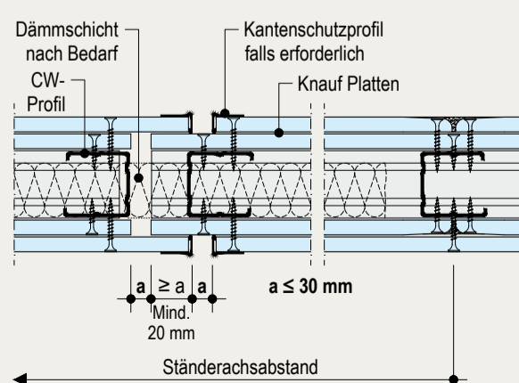
Bewegungsfuge ohne Brandschutz
