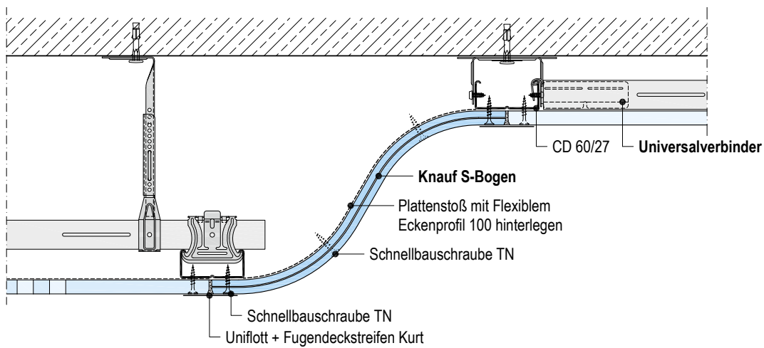
Flexibles Eckprofil
