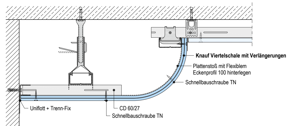
Flexibles Eckprofil
