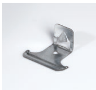
Συνδετήρας T για CD 60/27 Για εγκάρσια σύνδεση των οδηγών CD σε γωνία 90°.
