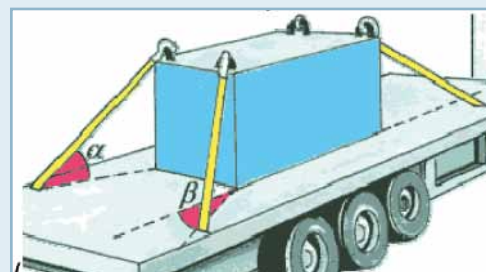
Πλευρική -/ Διαγώνια πρόσδεση με τις γωνίες \alpha και \beta
