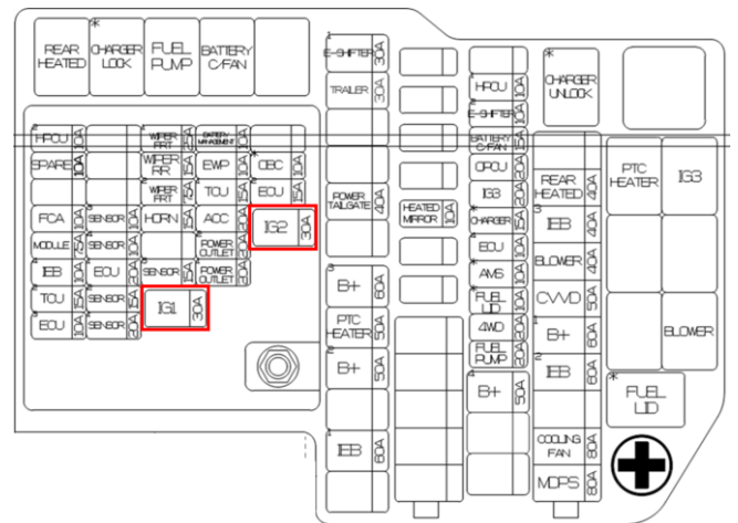
Caja de fusibles del compartimento del motor
