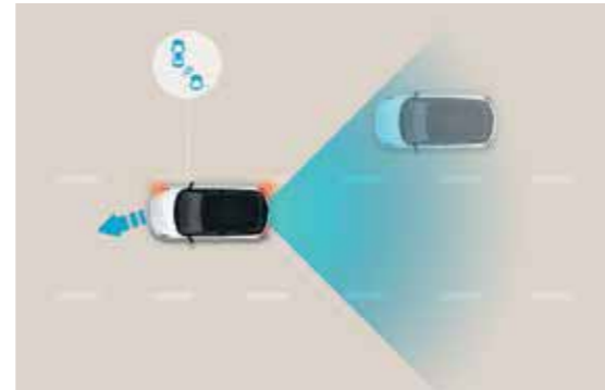
Blind-Spot Collision-Avoidance Assist (BCA) Door middel van radarsensoren in het onderste deel van de achterbumper en een camera vooraan waarschuwt dit systeem je voor verkeer in je dode hoek. Als je in een dergelijke situatie de richtingaanwijzer inschakelt, weerklinkt er een geluidssignaal en remt het systeem af om een aanrijding te vermijden.
