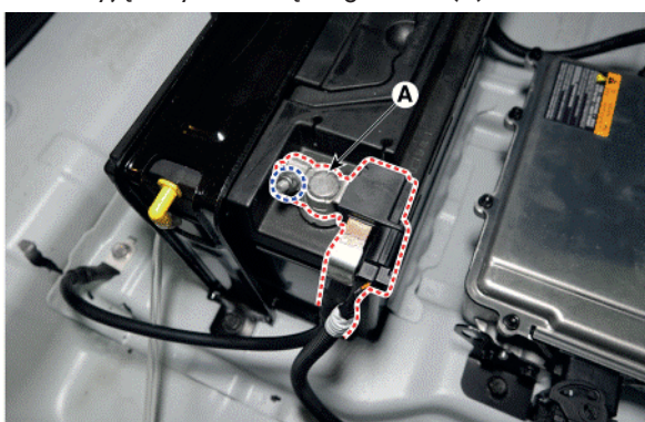
4-3. Wyłączyć stacyjkę (stan OFF) i odłączyć zacisk ujemny (-) (A) akumulatora 12 V.
