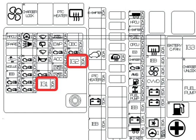
Skrzynka bezpieczników w przedziale silnika
