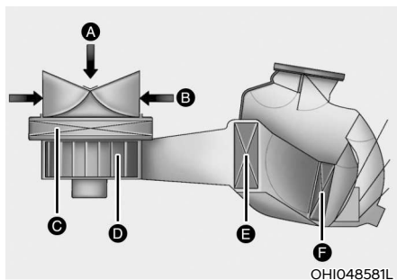
[A]: Vnější vzduch, [B]: Recirkulovaný vzduch [C]: Vzduchový filtr klimatizace, [D]: Ventilátor [E]: Jádro výparníku, [F]: PTC a vnitřní kondenzátor
