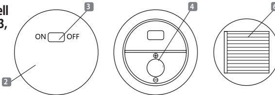
2 Batteriefach mit Solarpanel 3 Schalter (ON - OFF) 4 Batterie 5 Schrauben 6 Solarpanel
