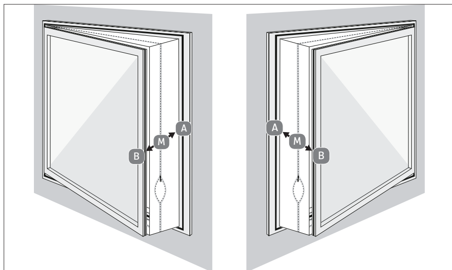
Fig. 12 – Montage sur fenêtre basculante
