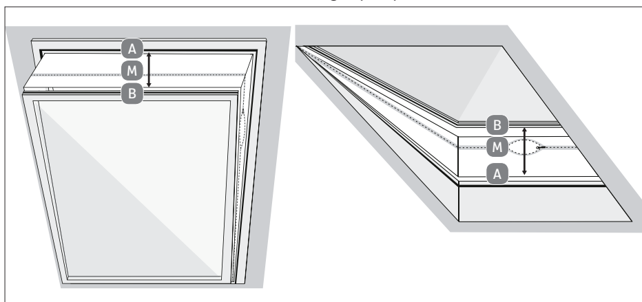
Afb. 13 – Montage op dakraam
