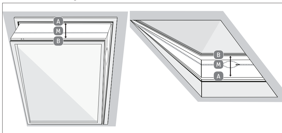
Fig. 13 – Instalación en ventanas de buhardilla
