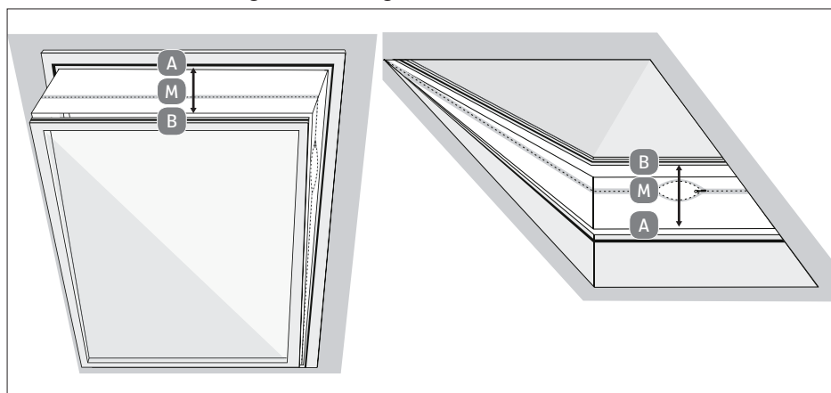
Fig. 13 – Montage sur fenêtre de toit
