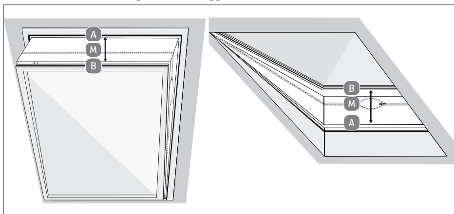
Fig. 13 – Montaggio su lucernari
