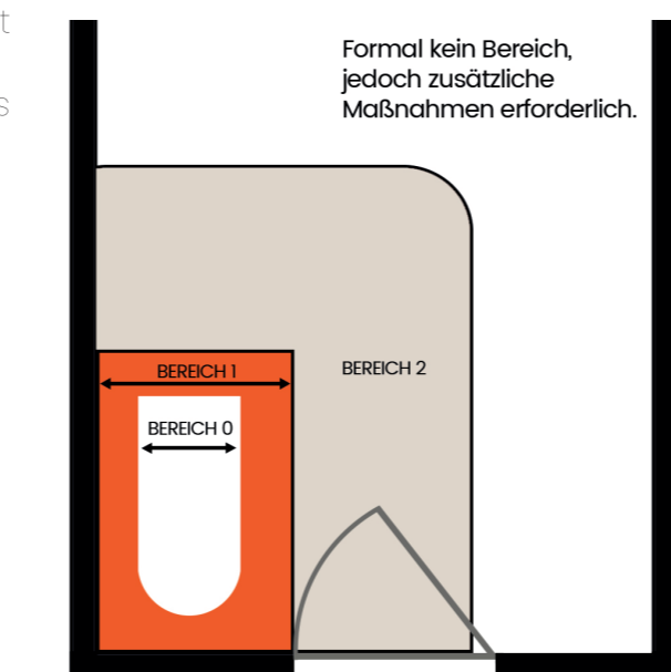
Abb. 02: Montage in Feuchträumen und Badezimmern
