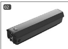
02 Batteria Inside (36V: 10/15/20 Ah 48V: 10/15 Ah)
