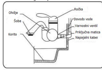
Zidna montaža
