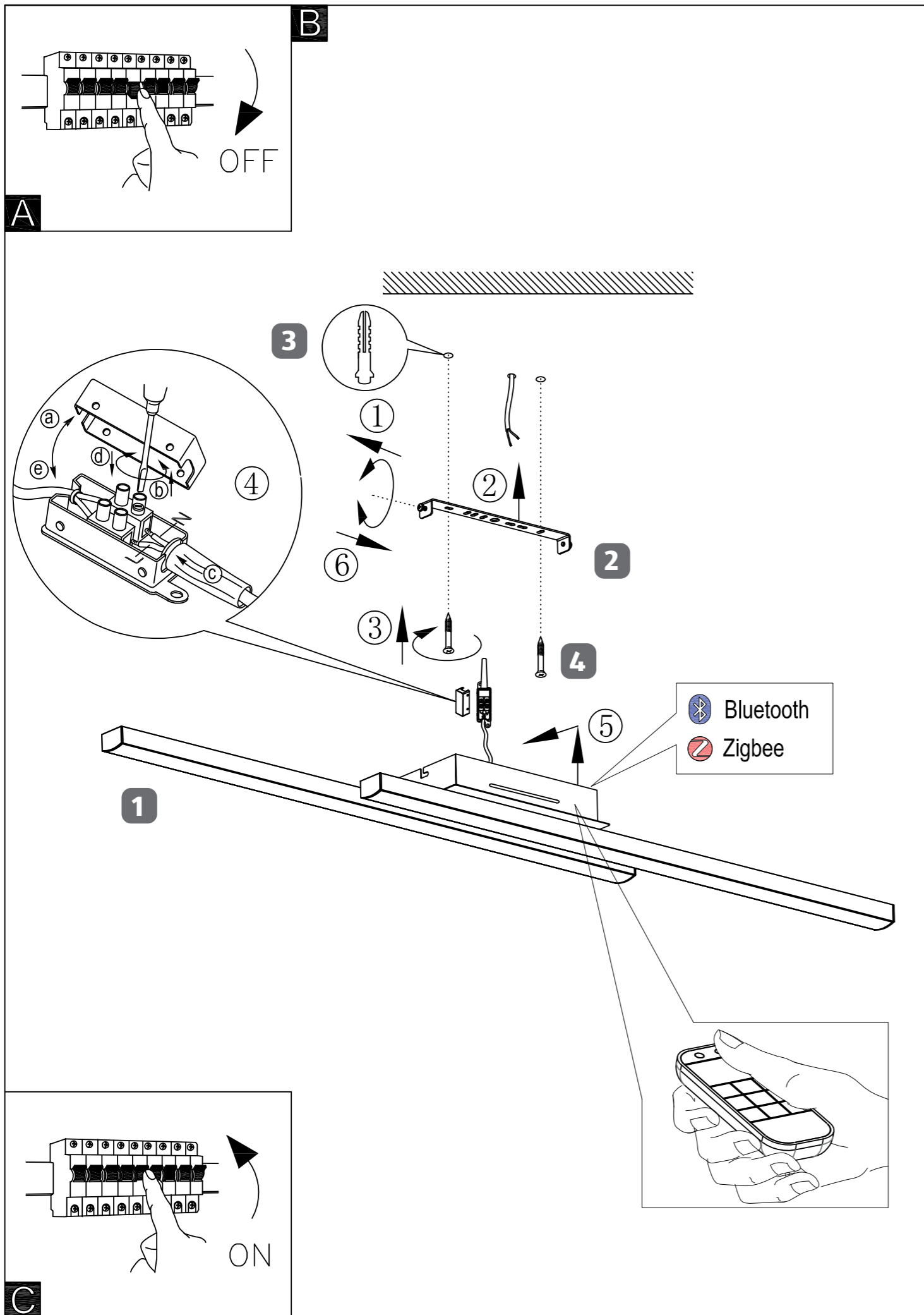
(Abb. 5) Fernbedienung
