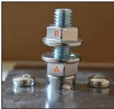
Abb. 05: obere Gewindebolzen
